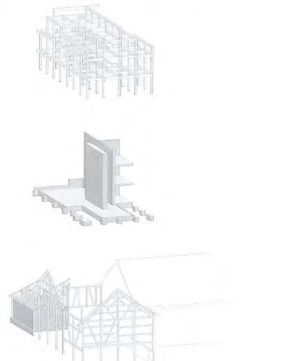
Nachdem die Betonelemente (Mitte) in den sanierten Bestand (unten) eingebaut wurden, folgte die Tragkonstruktion aus Holz.
